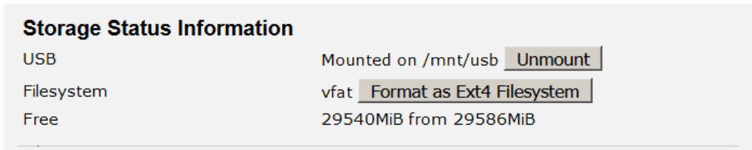
Abbildung 3.2: USB-Speicherstatus
