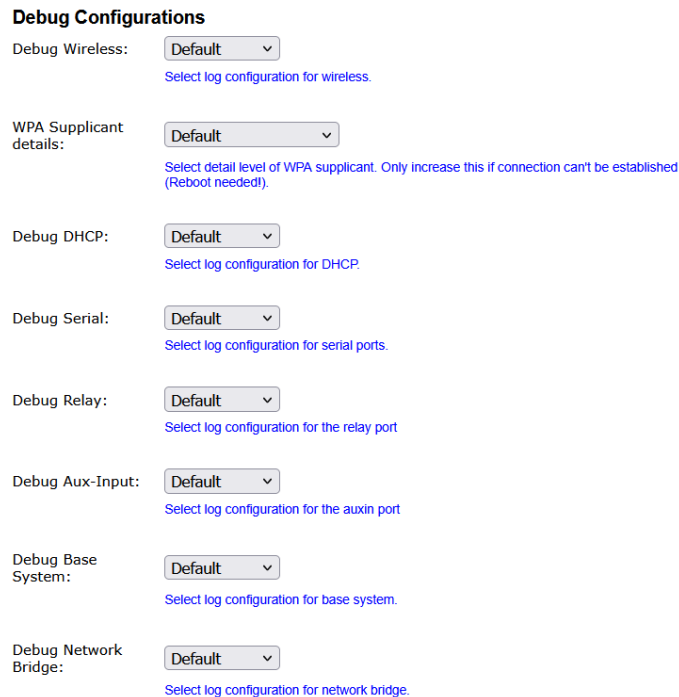
Abbildung 5.15: Debug Configurations
