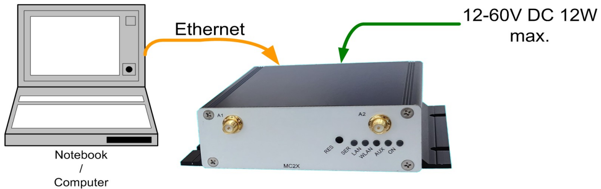
Abbildung 6: Aufbau zur Inbetriebnahme des MCX8
